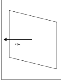
Figura 1.26: Vector en la dirección perpendicular a esta página.
