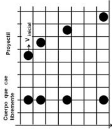
Figura 2.52: Posiciones para tiempos iguales de dos objetos, uno en caída libre y otro con movimiento de proyectil.
