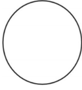
Figura 2.17: Trayectoria circular.
