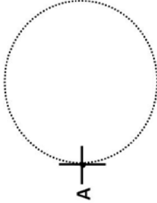
Figura 2.13: Una vuelta completa, comienza en el punto A y termina en el punto A.
