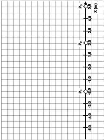
Figura 2.6: Puntos sobre una línea recta
