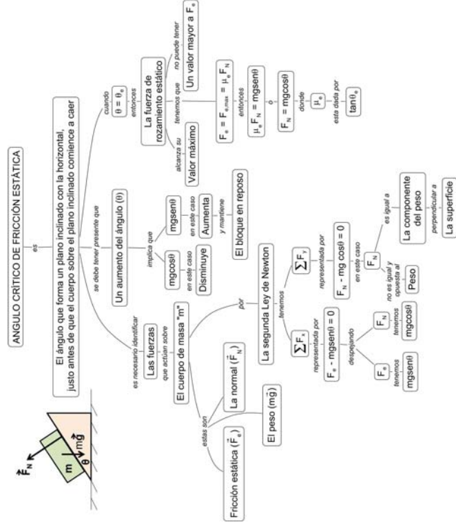
Figura 3.19: Ángulo crítico.
