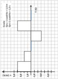
Figura 2.31: Gráfica velocidad vs tiempo.
