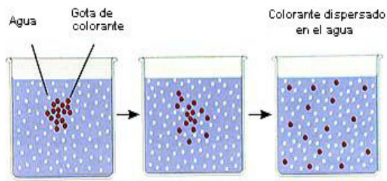
Fig. 4. Difusión
