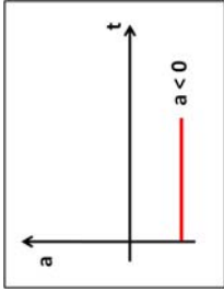
Figura 2.42: Gráfica aceleración vs tiempo.
