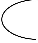
Figura 2.19: Trayectoria parabólica.
