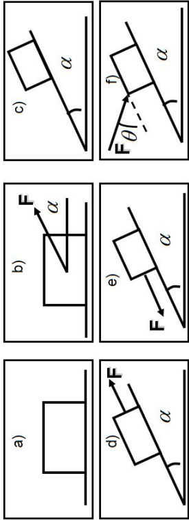
Figura 3.20: Identificar las fuerzas que actúan sobre los cuerpos.
