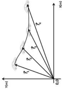
Figura 2.16: Trayectoria de un automóvil en movimiento.
