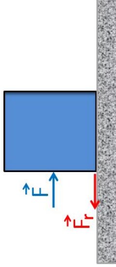
Figura 3.16: La fuerza de fricción se opone al movimiento.
