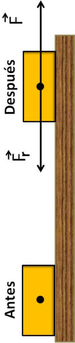
Figura 3.7: La fuerza como causa del cambio de movimiento de los cuerpos.
