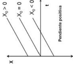
Figura 2.26: Pendiente positiva de la velocidad.
