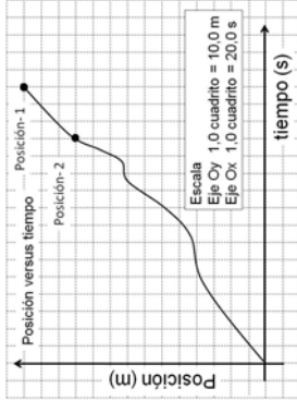
Figura 2.24: Representación gráfica de un cuerpo cuyo movimiento es variado a lo largo del tiempo.
