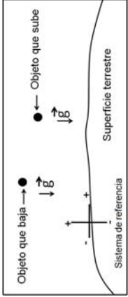
Figura 2.50: El sentido de la gravedad, asunto de convención.
